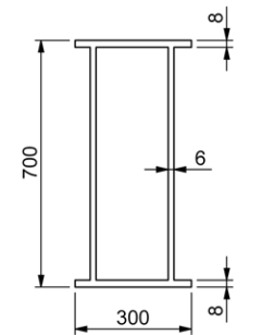
Mặt cắt dầm chính
